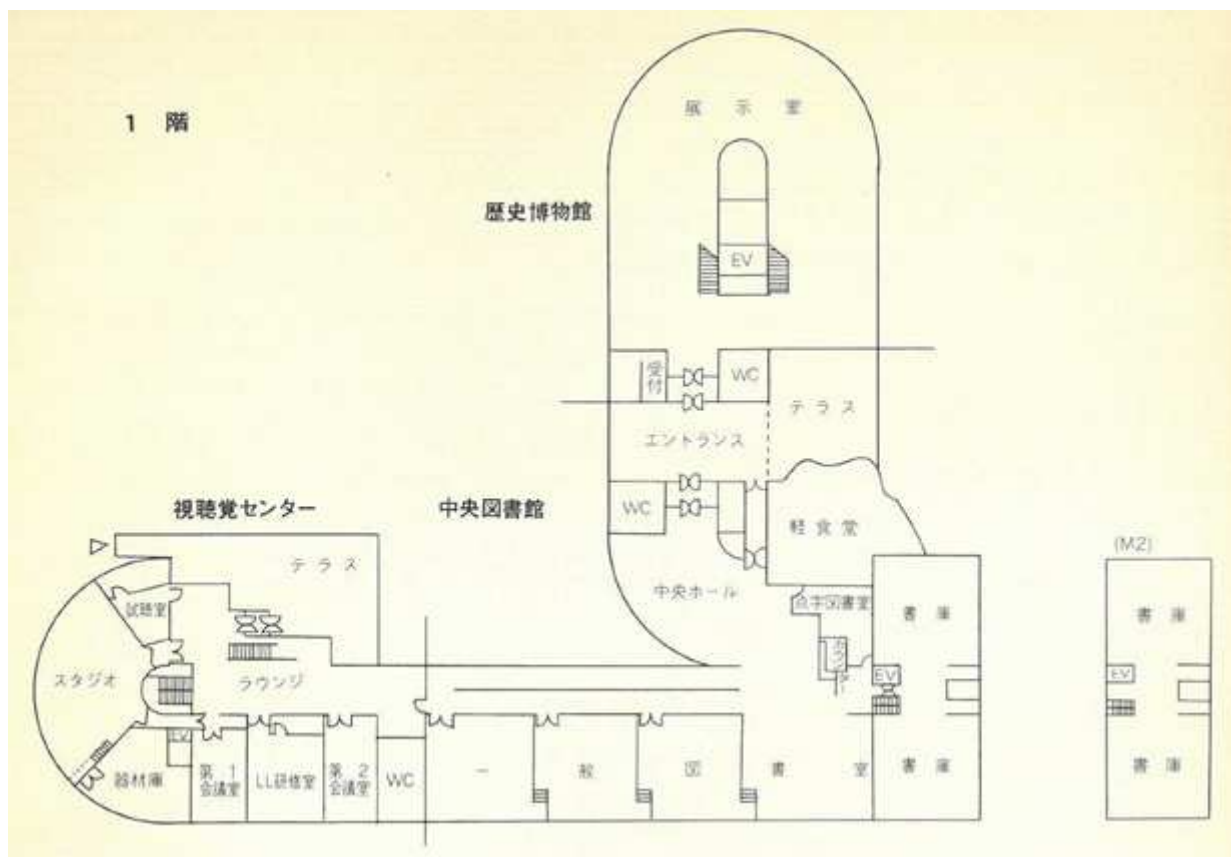
平面図（1階）
